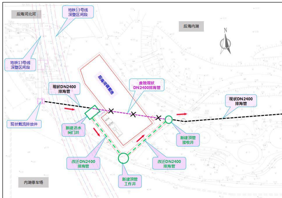
图 2.6-2 排海管现状废除示意图
