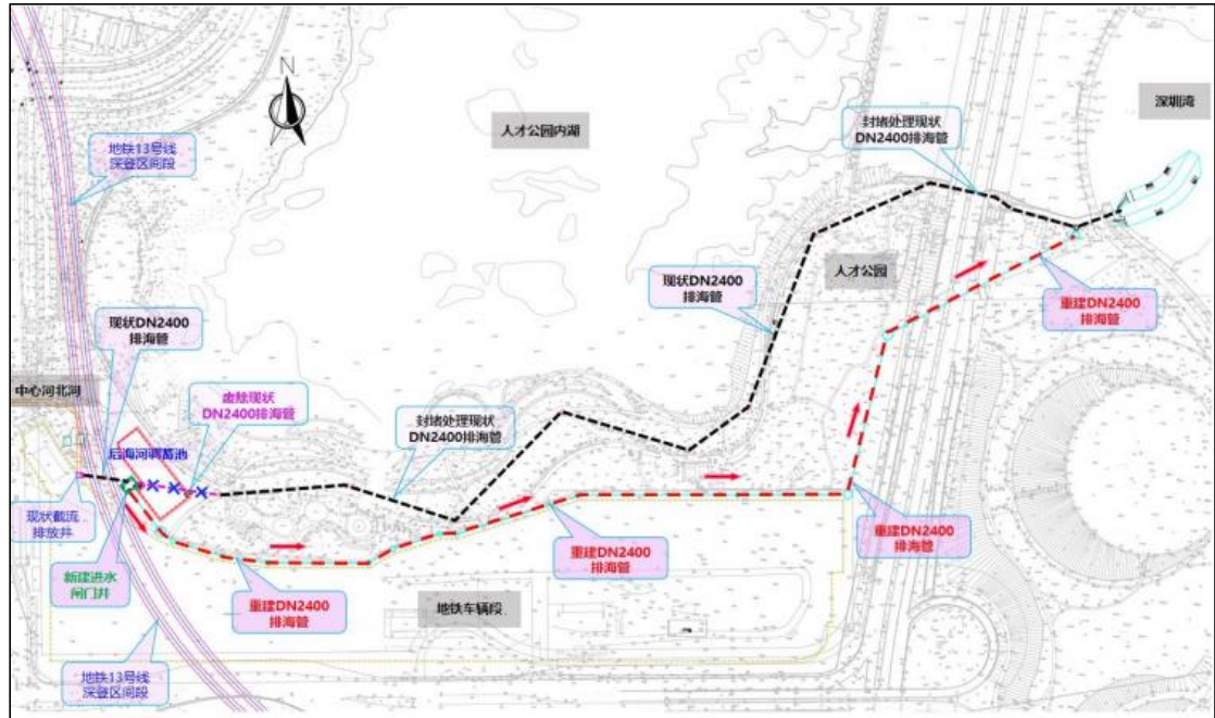
图 2.6-1 明挖+顶管方案平面图
