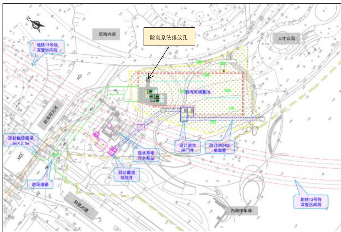
图 2.5-2 调蓄池总平面布置图
