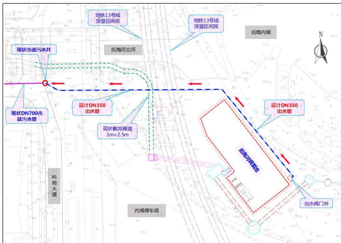
图 2.5-7 调蓄池出水方案平面图
