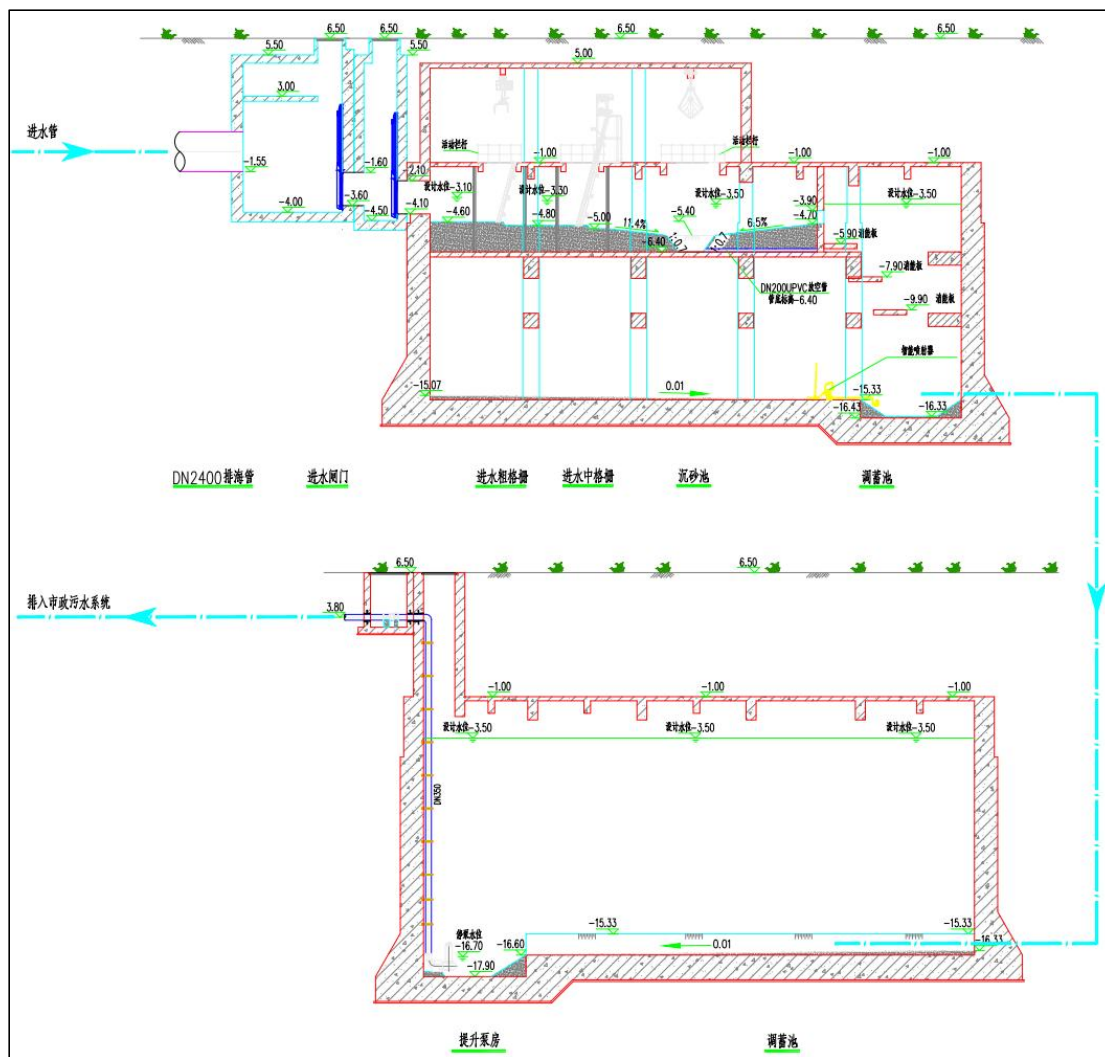
图 2.5-8 调蓄池工艺流程图
