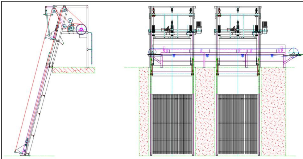
图 2.5-11 中格栅大样图
