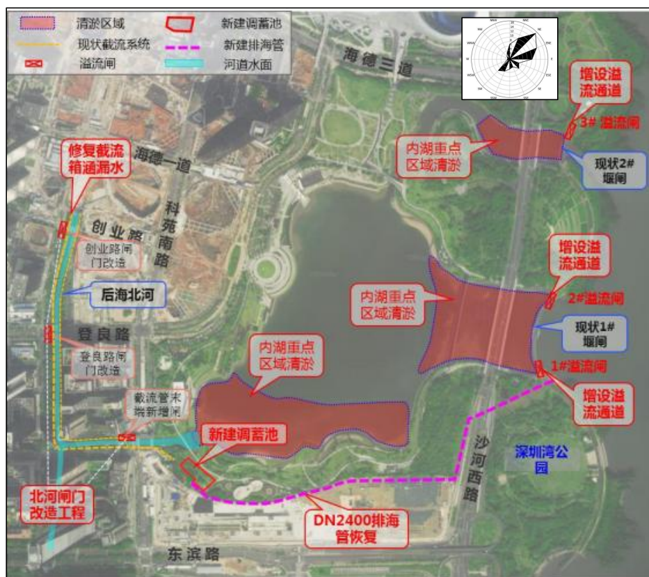
图 2.1-1 工程总体布局图
