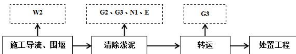
图 3.1-3 清淤工程施工工艺及产污环节
